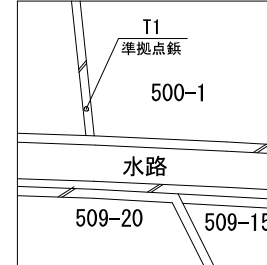
準拠点位置詳細図
