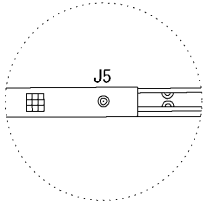
引照点詳細図(J5) S=1:250
